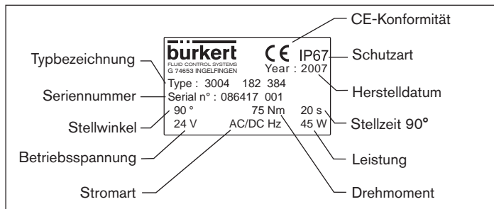
Bild 4: Beschreibung des Typenschildes
