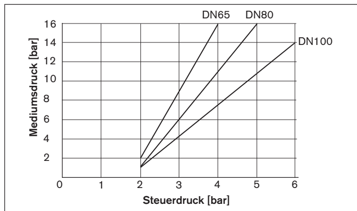
Bild 5: Druckdiagramm, Steuerfunktion B und I, Anströmung unter Sitz
