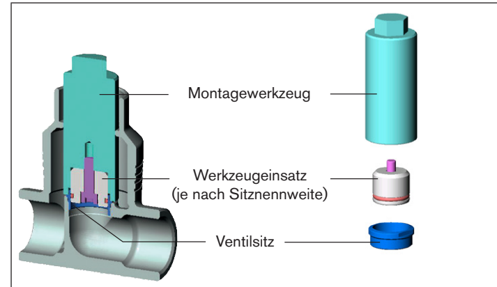
Bild 7: Austausch des Ventilsitzes
