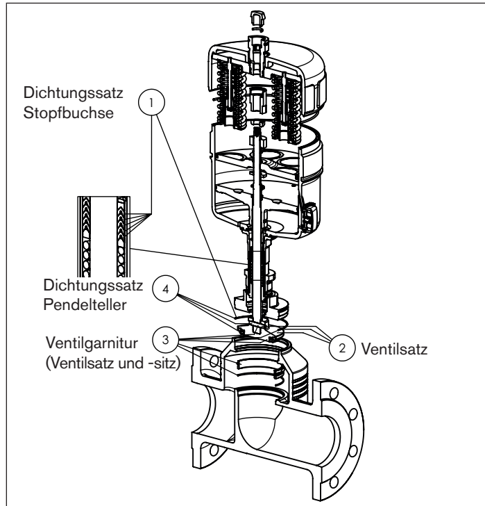
Bild 8: Übersicht Ersatzteilsätze
