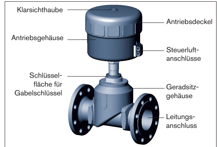
Bild 1: Geradsitzventil Typ 2012, Aufbau und Beschreibung
