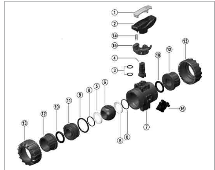
Fig. 2 : Vue éclatée du modèle 3 voies du robinet à bille synthétique
