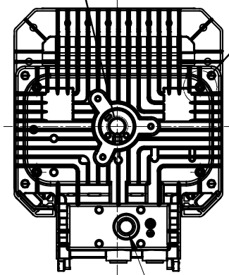
VUE ARRIÈRE
